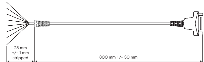
Cable - CU-0.8M-BK-WO.PL-SYS.PL (538745)
