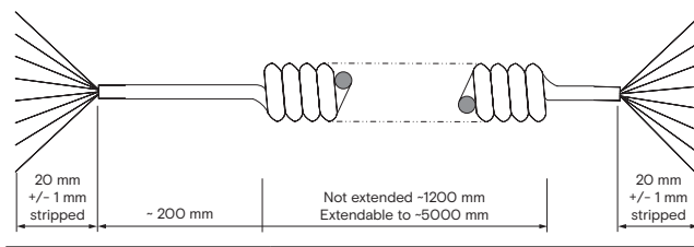
Cable - H1200-5000 (1000457)
